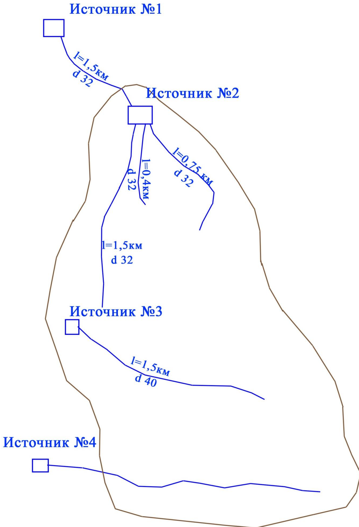
Схема водопроводных сетей в селе Аялизимахи
